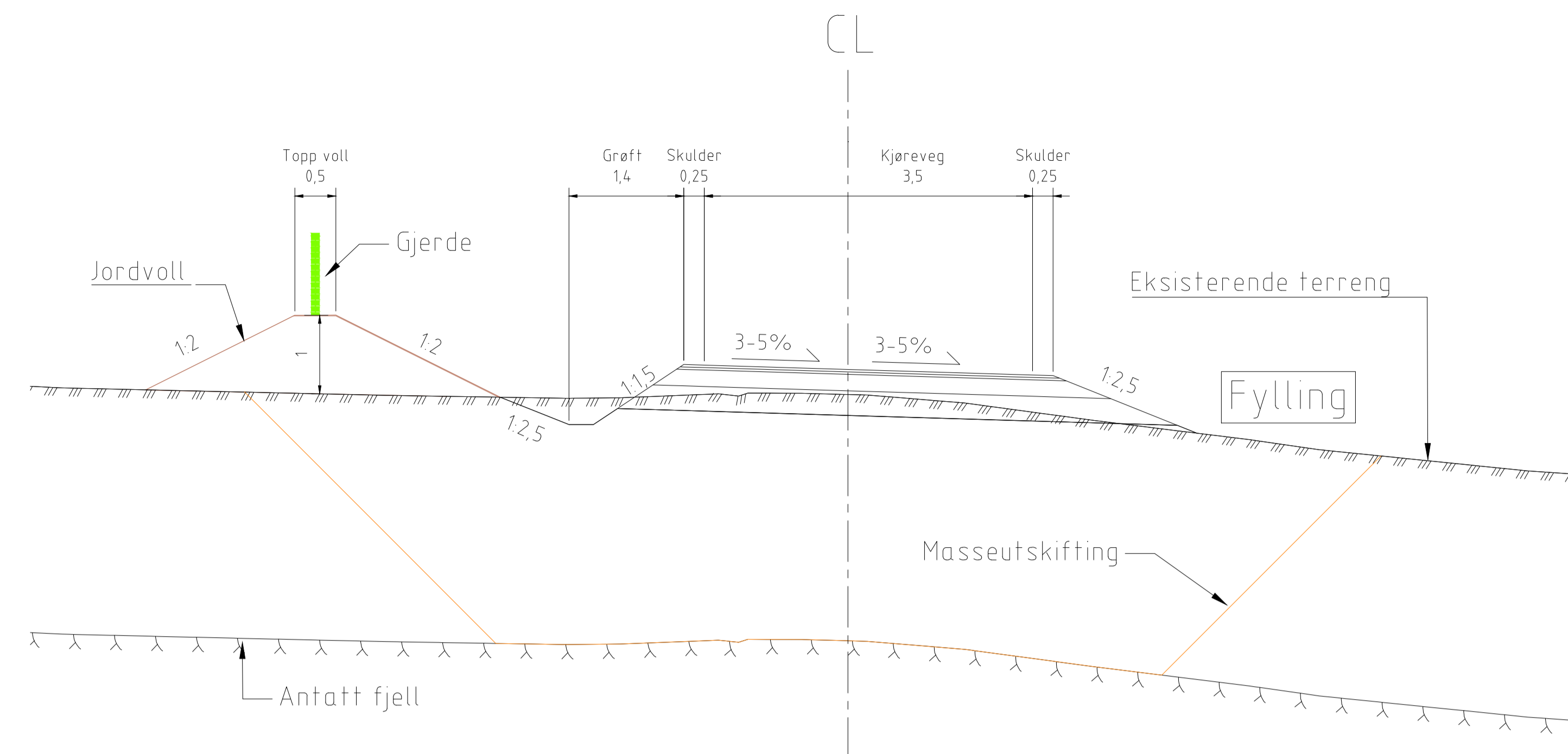
NORMALPROFIL* Veg 20 000 Voll med rekkverk
