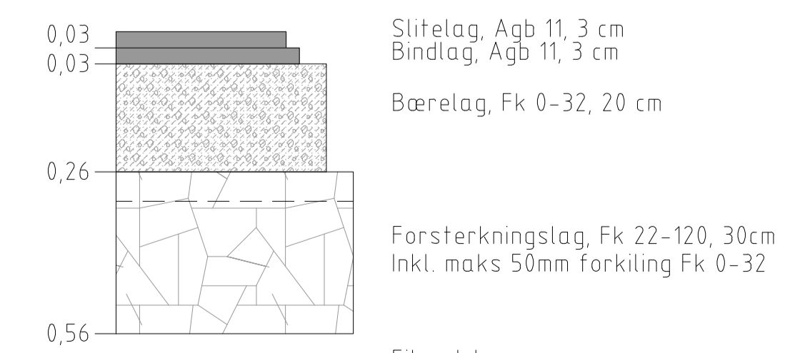
Eksisterende underbygning
