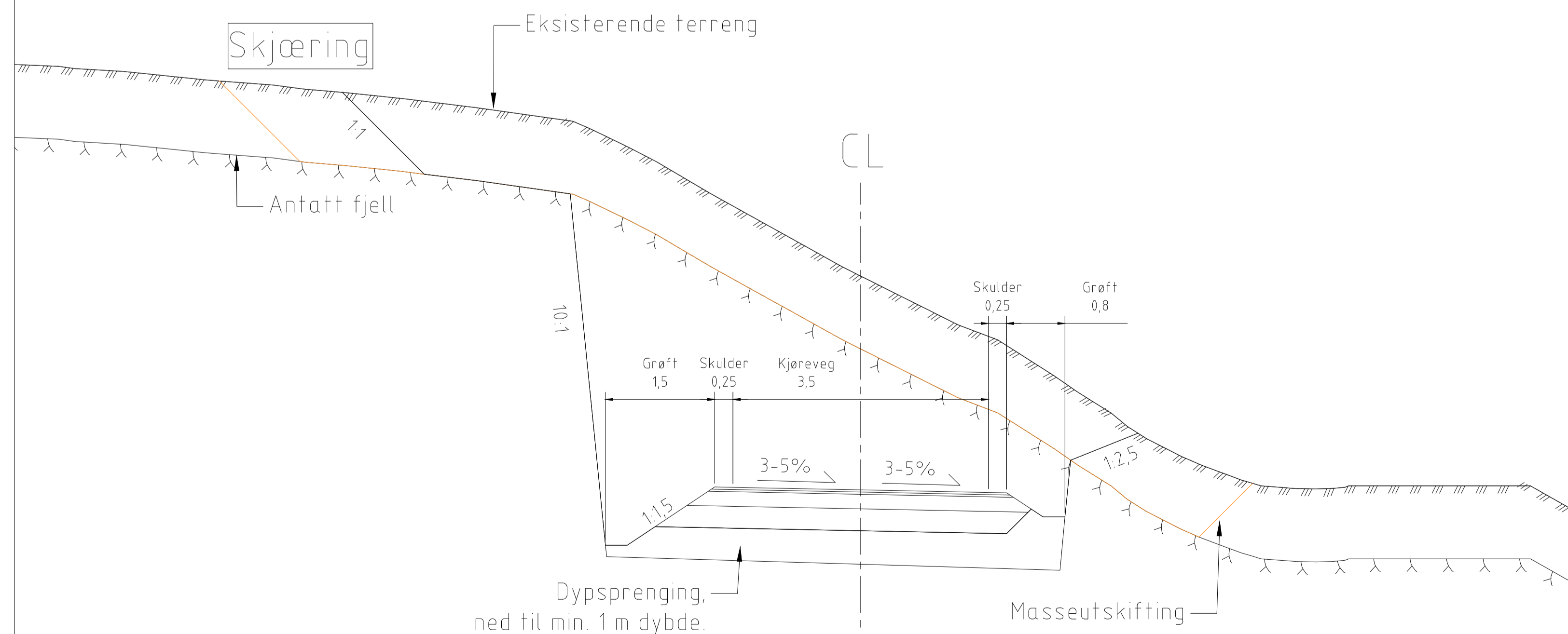
NORMALPROFIL Veg 20 000 Overbygning i fjell
