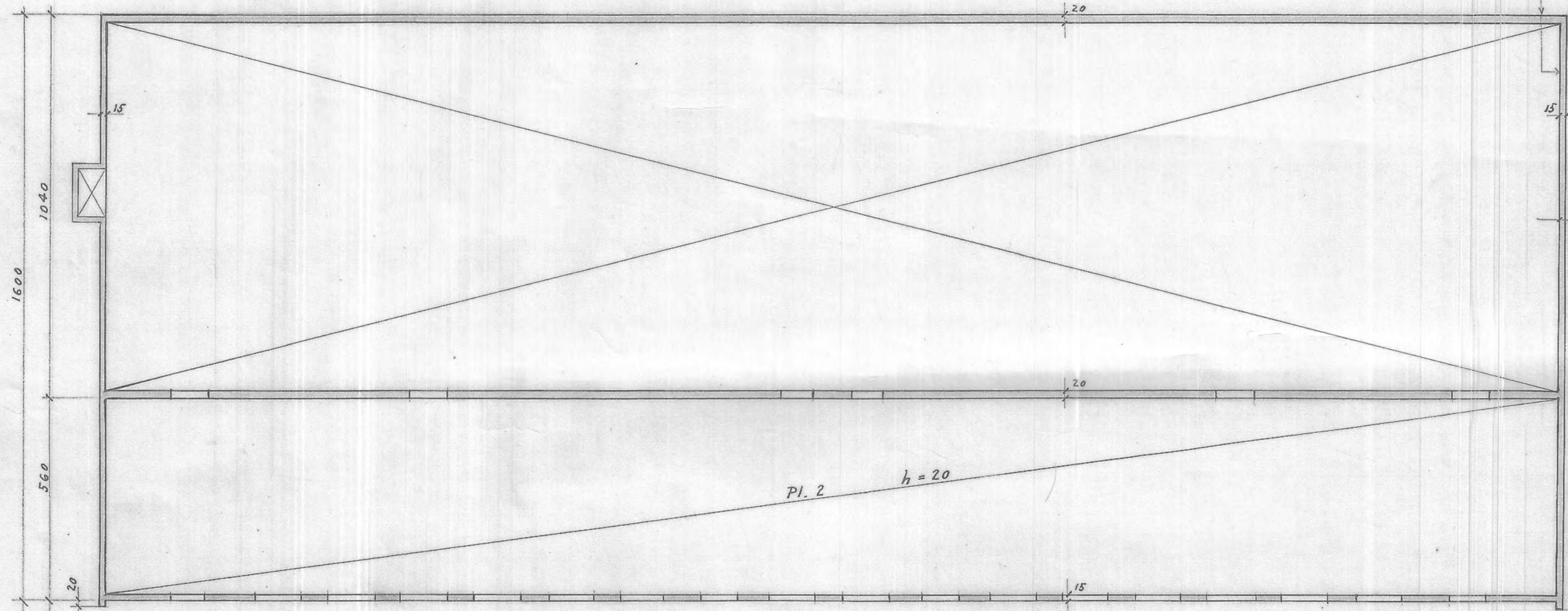
Plan Nedre tak.
