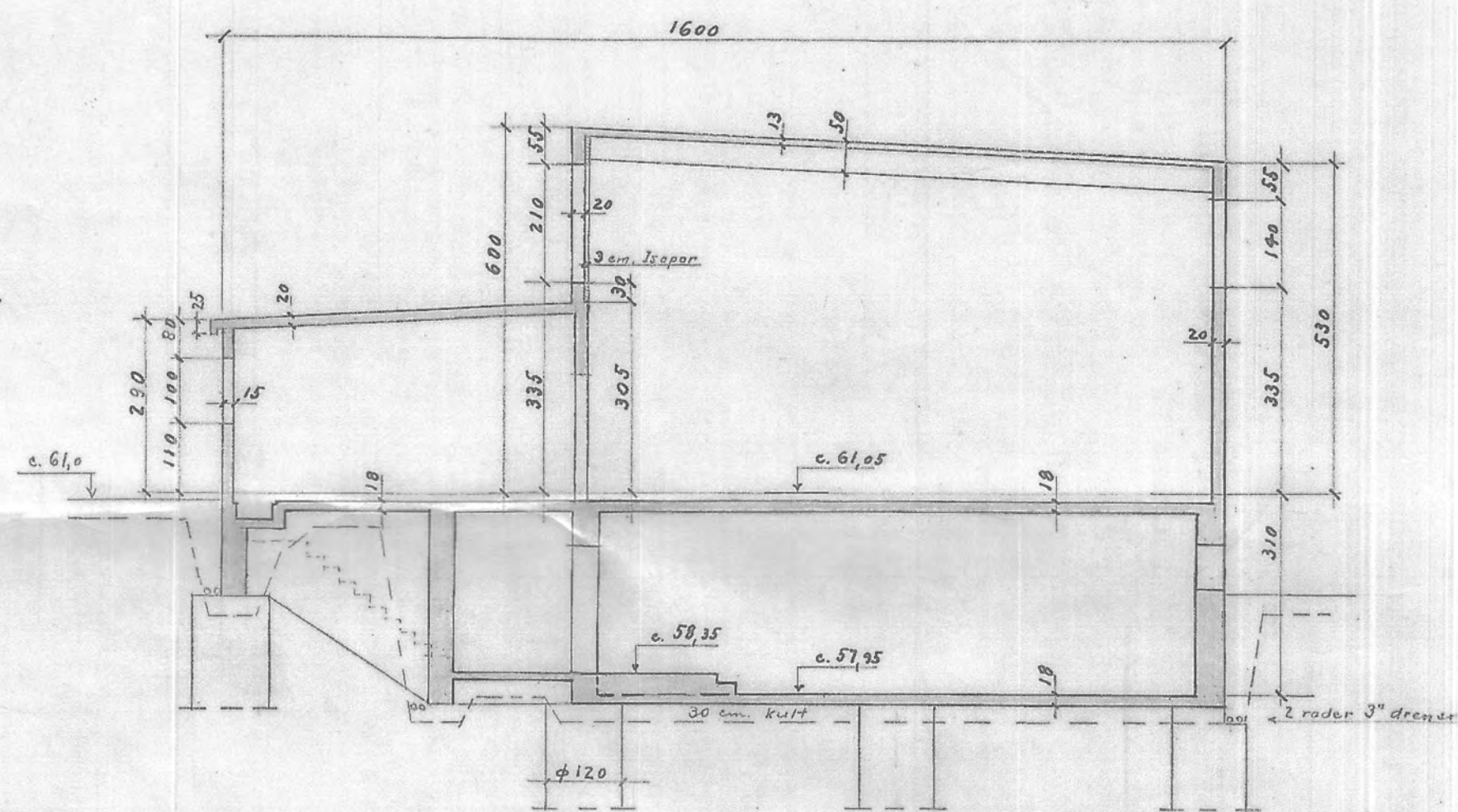
Snitt A-A
