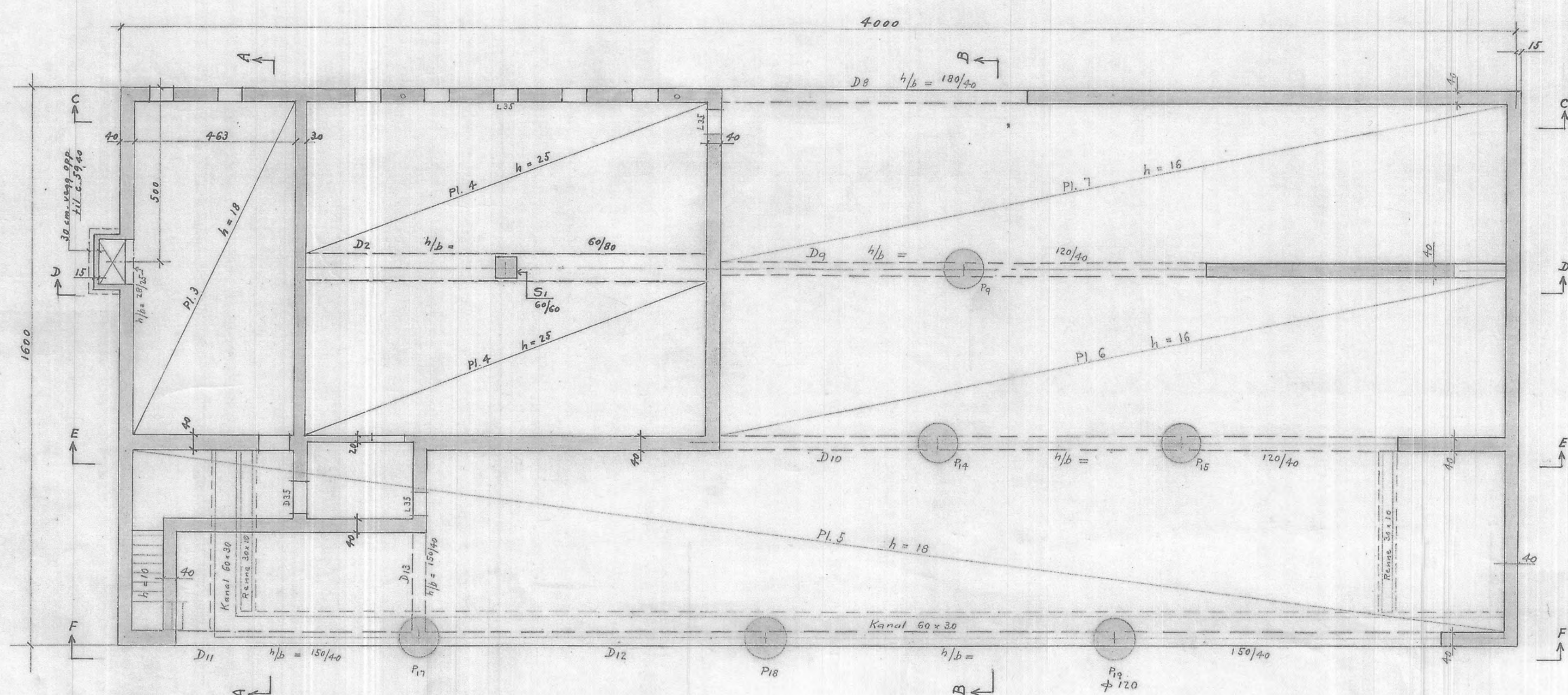
Gulv i 1. etasje. Vægger i tilfluktsrom og fyrrum. Fundamentvegger og -pilarer.
