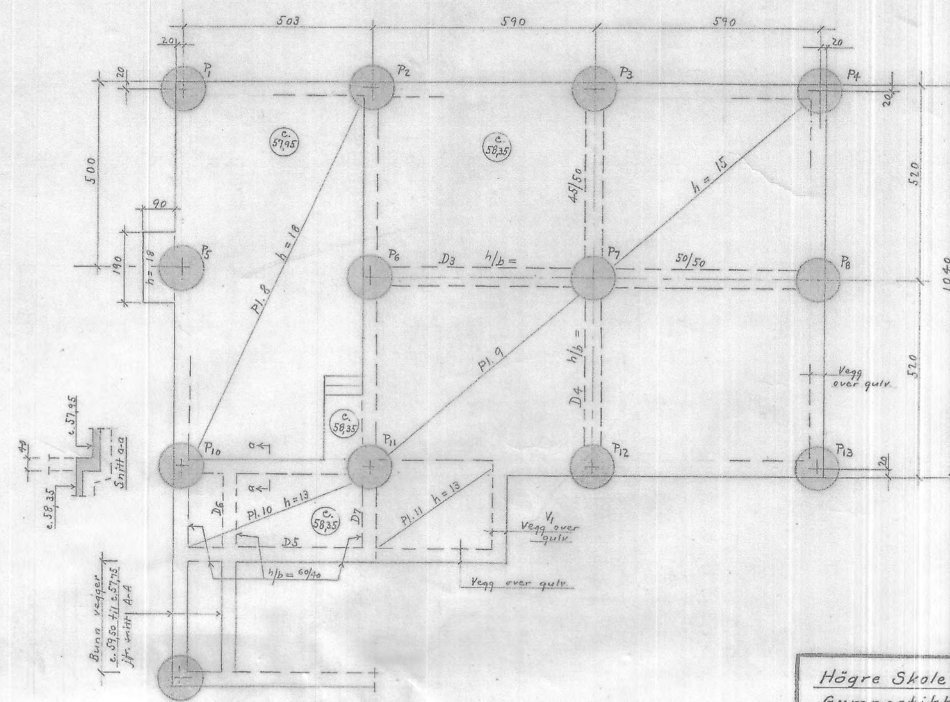
Gulv i tilfluktsrom og fyrrum. Fundamentpilarer.
