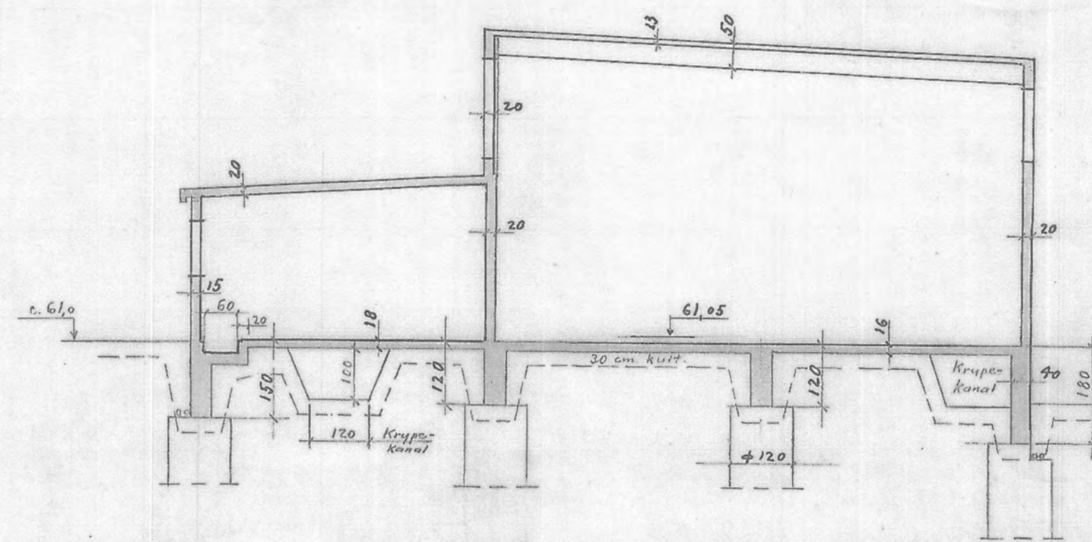
Snitt B-B
