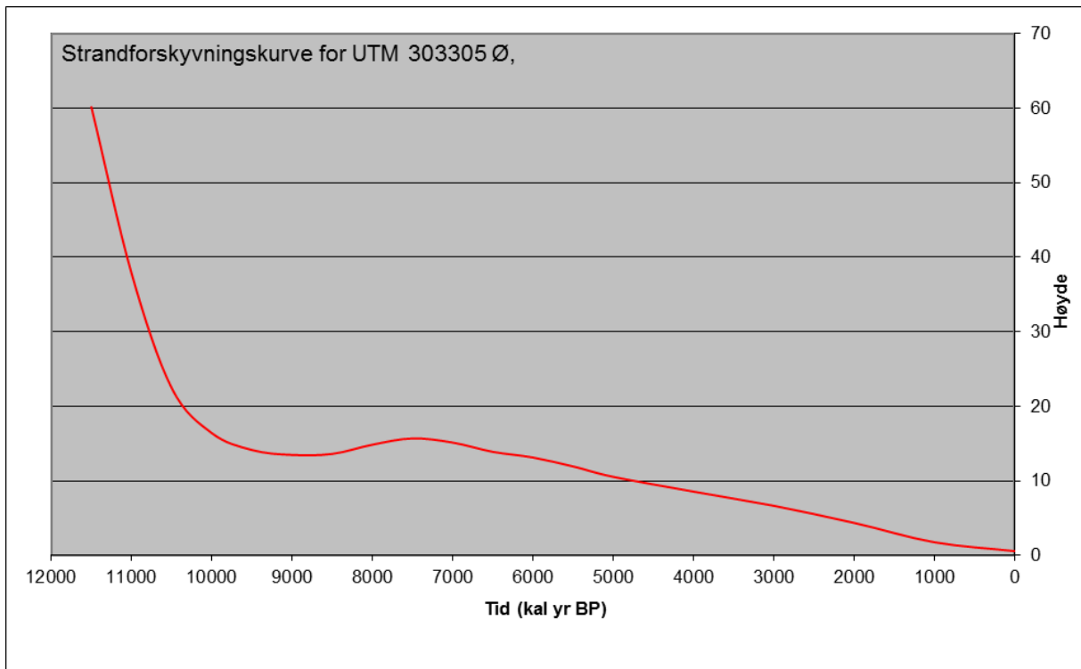
Figur 1. Strandforskyvningskurve for Arna, Bergen kommune.
