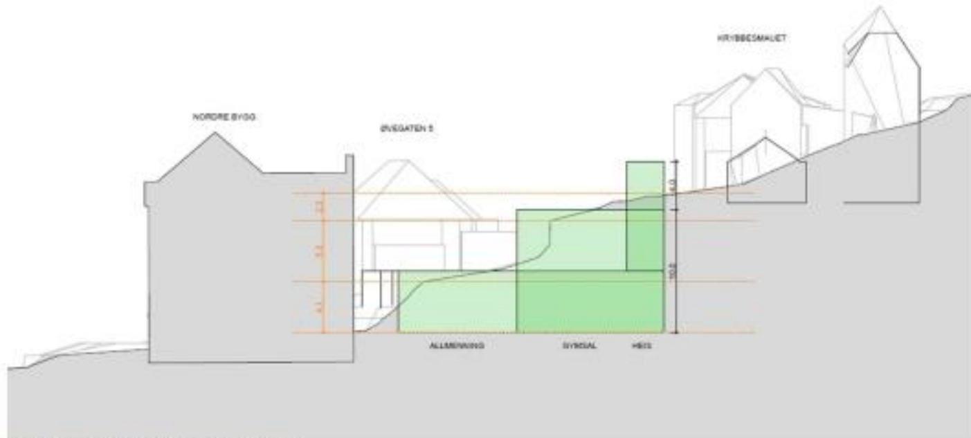
Figur 15 Alt. K2 utvidelse, terrengsnitt.
