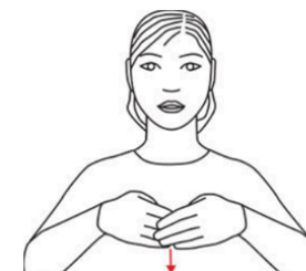
Venn
