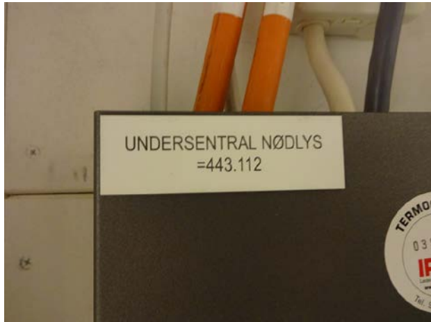
Eksempel på merking av en undersentral i systemet for nødlys.
